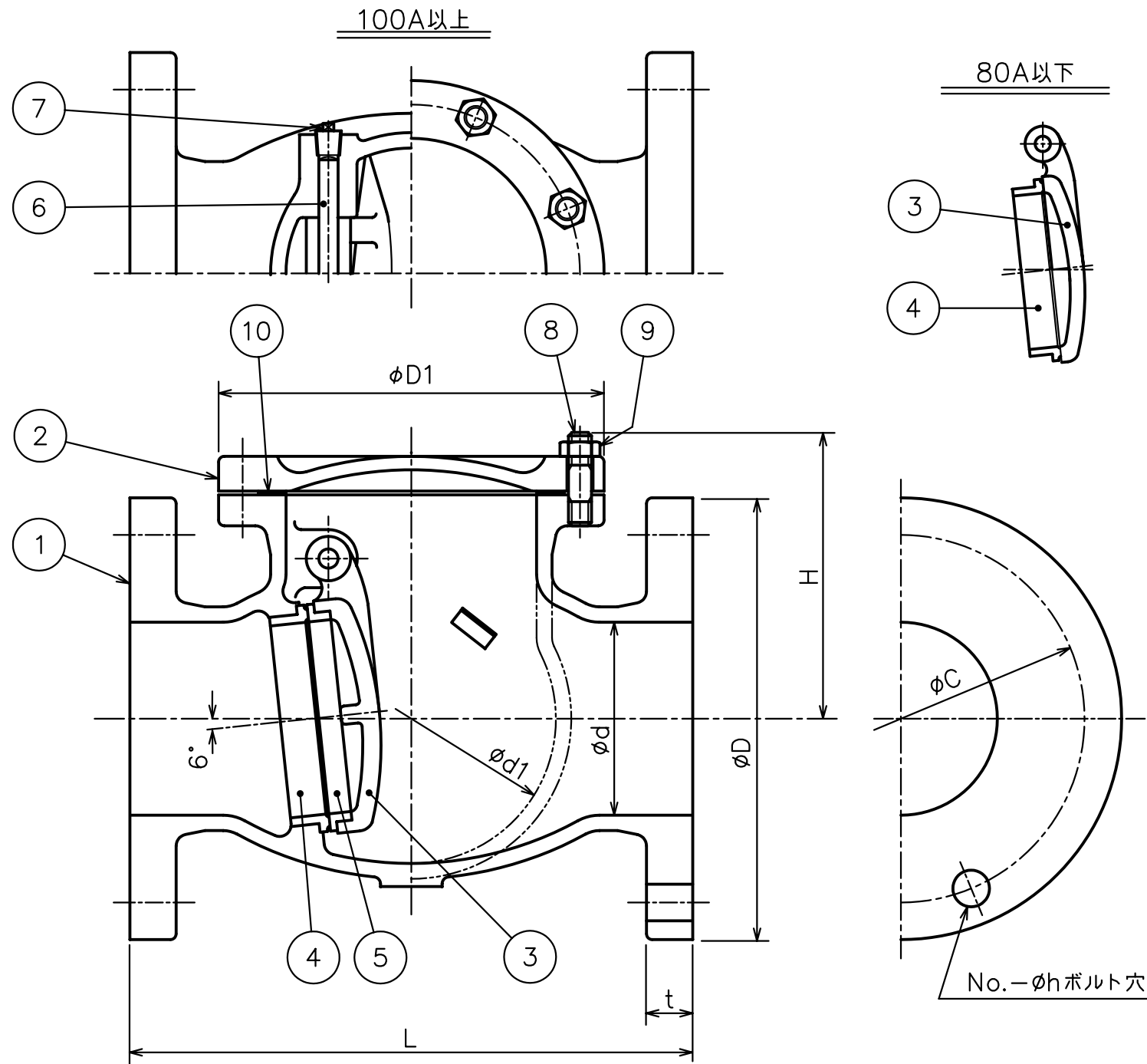
フランジ：JIS B2239 10K
